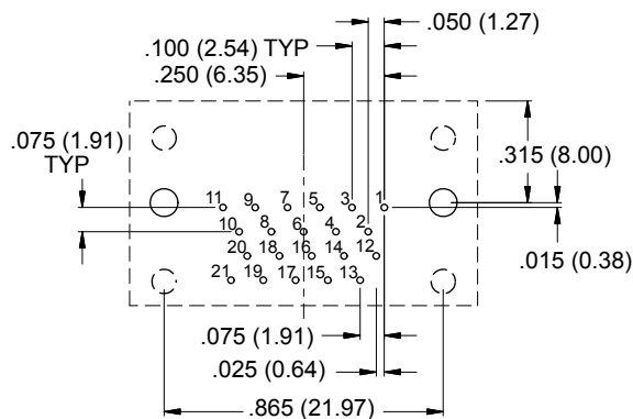
21 SOCKET
