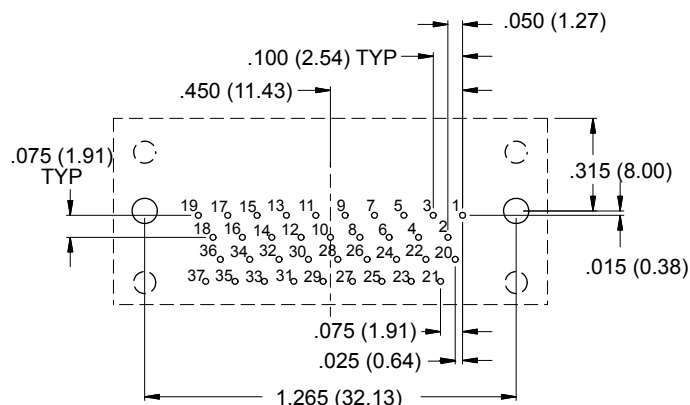
37 SOCKET
