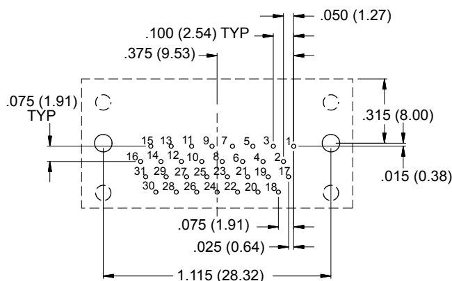
31 SOCKET
