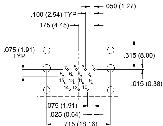
15 SOCKET
